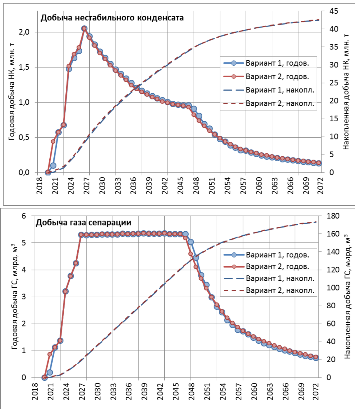
Рисунок 3. Сопоставление графиков добычи углеводородов по вариантам разработки, участок 4А.
