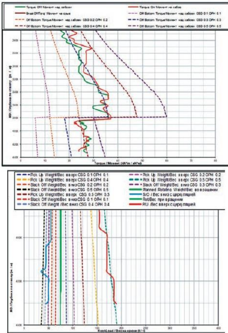
Рисунок 5 – Графики крутящих моментов и веса на крюке показывающие anomalно высокие значения.
