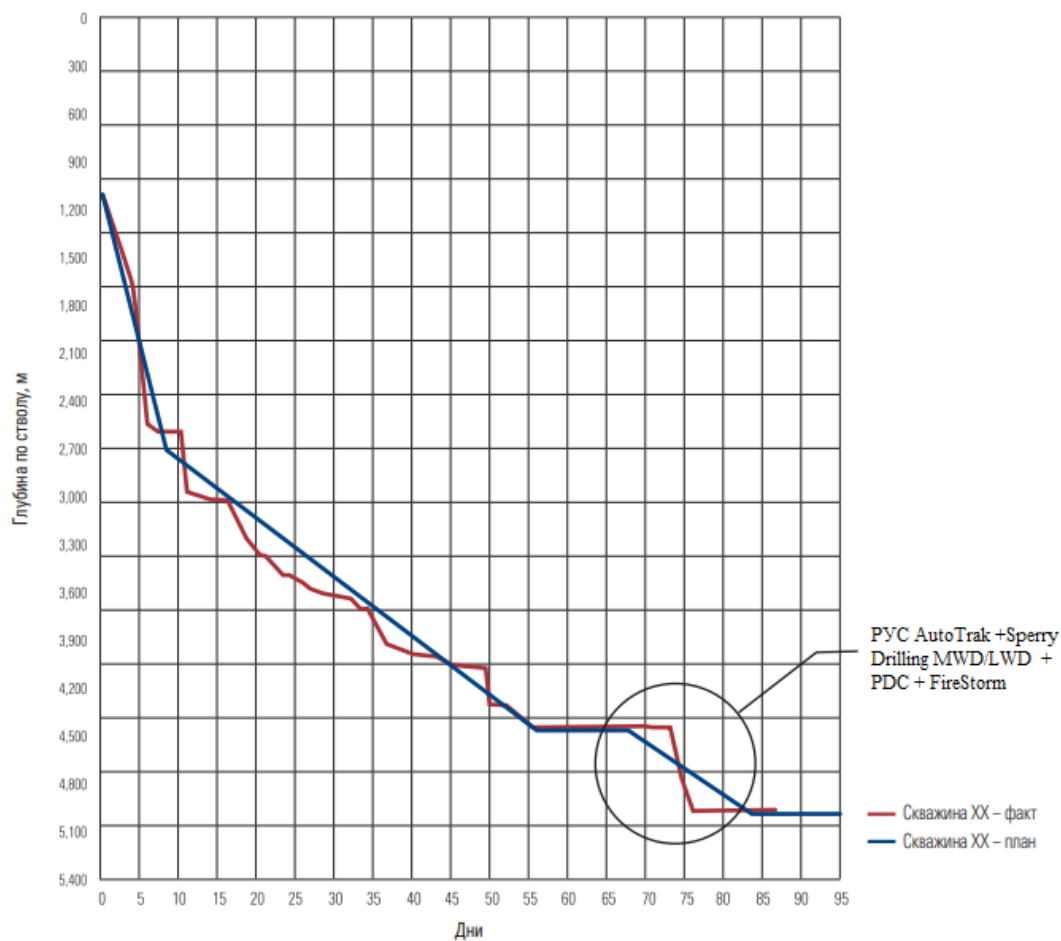
Рис. 2 - Бурение бокового ствола на скважине №6892 с интенсивность набора зенитного угла 10^\circ/30 м с использованием PDC AutoTrak +Sperry Drilling MWD/LWD +PDC FireStorm
