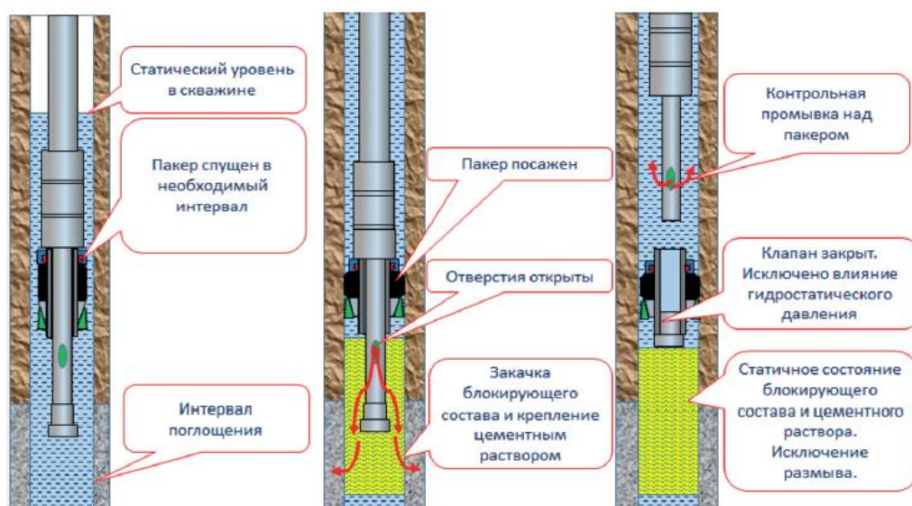
Рисунок 1 – План схема работ по изоляции зоны ухода промывочной жидкости
