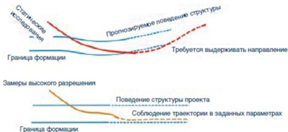
Рисунок 4 - Влияние применения замеров высокого разрешения TC Sperry Ssp на расположение трассы скважины.
