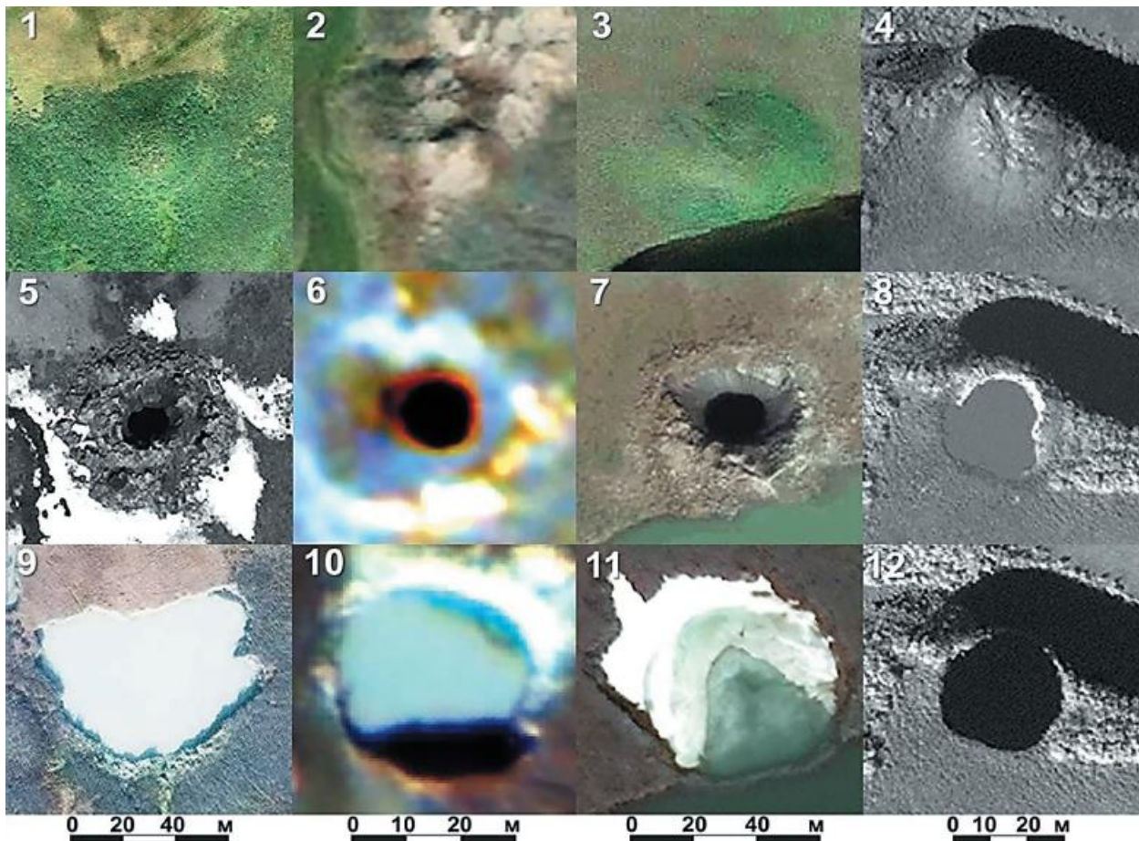
Рисунок 2. Многолетние бугры пучения в процессе своей эволюции
