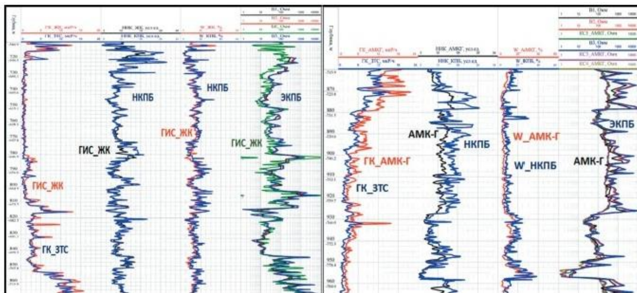
Рисунок 1 – Данные по модулям нейтронного и бокового электрического каротажа ТС «Геонавигация» ТНГ-Групп и Sperry San
