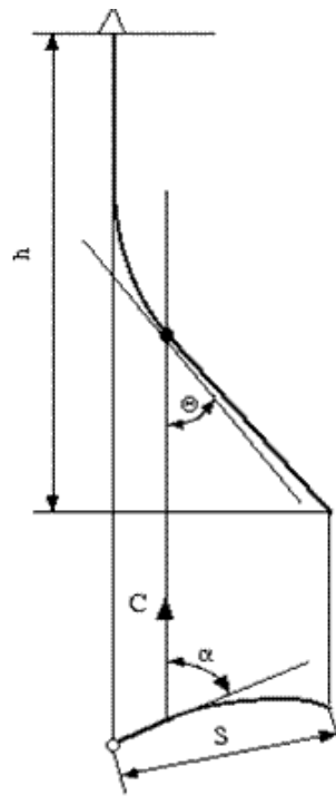
Рис. 1 – Элементы пространственного расположения скважины
