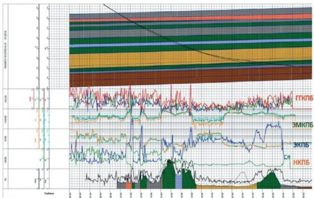
Рис. 2 . Минигеологическая модель
