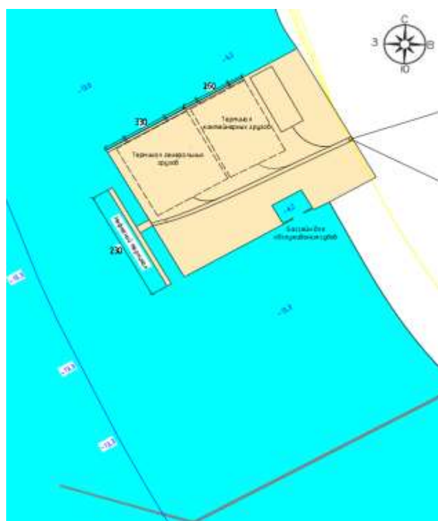
Рисунок 3. Мастер-план п. Корсаков – вариант 2
