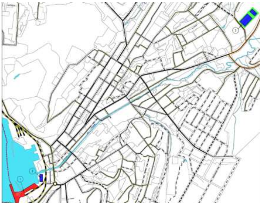
Рисунок 2. Мастер-план п. Корсаков – вариант 1
