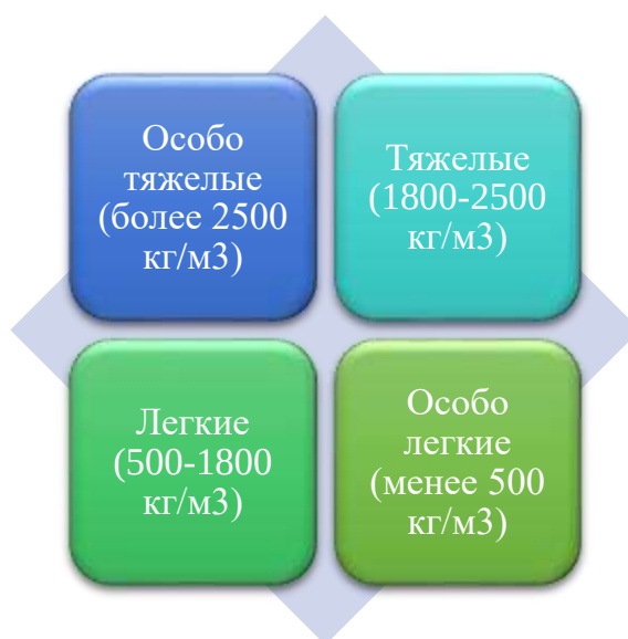
Рисунок 1 – Классификация бетона по плотности
